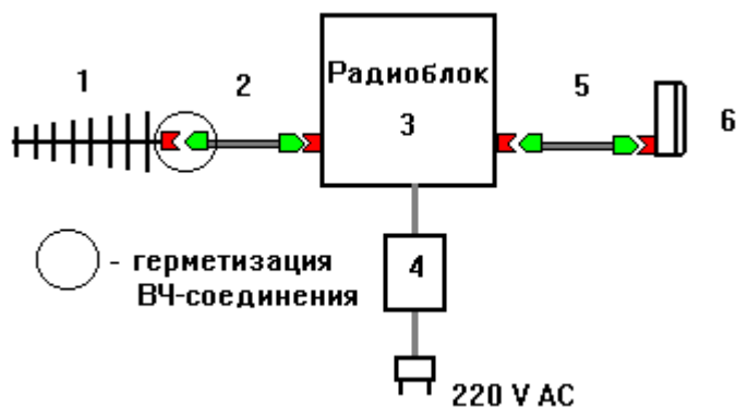
Рис. 2 Схема подключения ретранслятора
